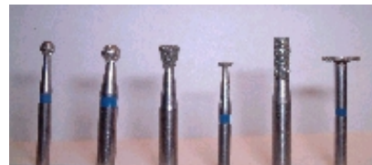
DIAMOND TIPPED BURRS 421D1 421D2 421D3 421D4 421D5 412D6
