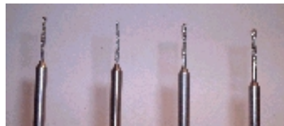
DIAMOND SPIRAL BURRS 558D8 (0.8mm) 558D9 (0.9mm) 558D10 (1.0mm) 558D12 (1.2mm)
